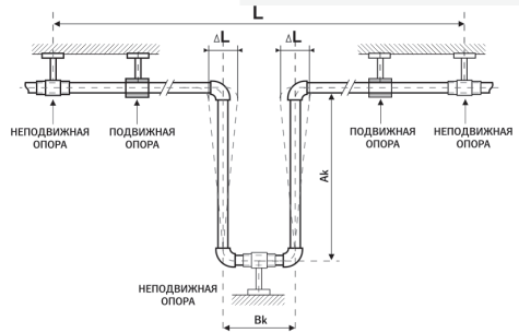
Рисунок 3. П-образный компенсатор
