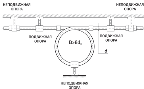
Рисунок 5. Петлевого компенсатор
