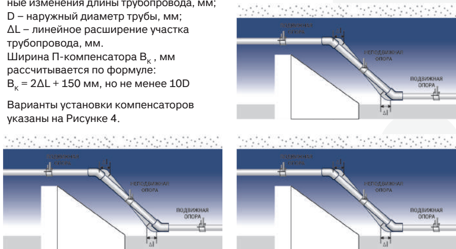
Рисунок 4. Варианты установки компенсаторов
