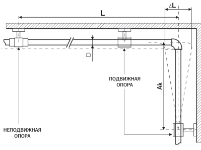
Рисунок 2. Г-образный компенсатор
