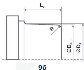
9б Рисунок 9. Сварочные насадки
