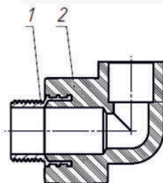
Рисунок 11. Комбинированный фитинг
