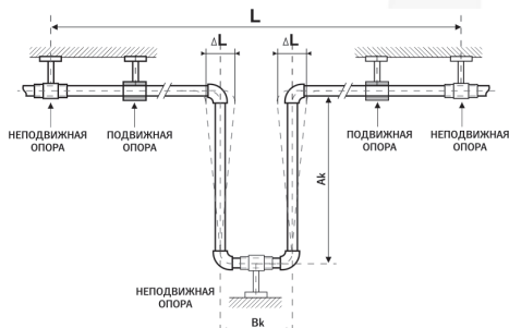
Рисунок 3. П-образный компенсатор
