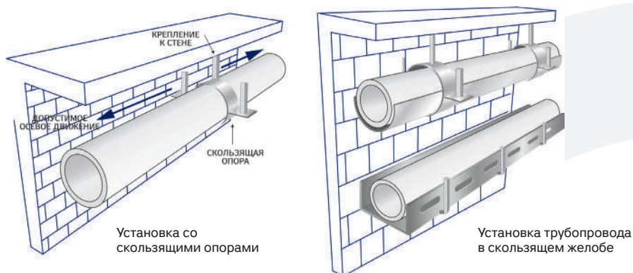
Рисунок 7. Крепление с подвижными опорами
