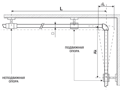
Рисунок 2. Г-образный компенсатор
