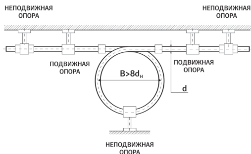
Рисунок 5. Петлевой компенсатор
