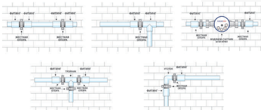
Рисунок 6. Крепление с жесткими опорами
